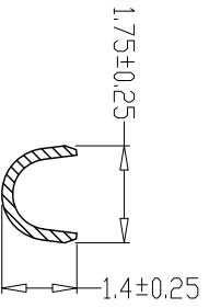
SEC:B-B
